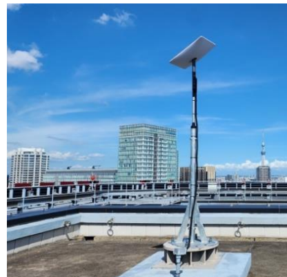
ビル屋上へのアンテナの設置風景
